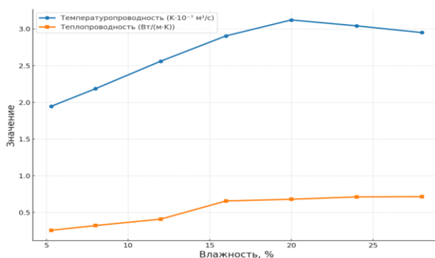
Рис.1. Изменение коэффициентов температуропроводности и теплопроводности сероземно-луговой почвы при плотности 1,3 г/см 3 в зависимости от влажности (W)
