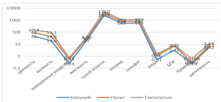
Рис. 1. Сравнительный анализ качества поверхностных вод в трёх зонах Республики Каракалпакстан по результатам весеннего мониторинга 2025 года.
