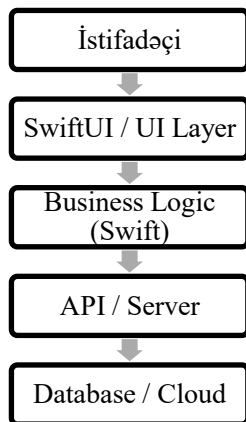
Sxem 1. iOS tətbiq arxitekturasında Swift-in yeri
